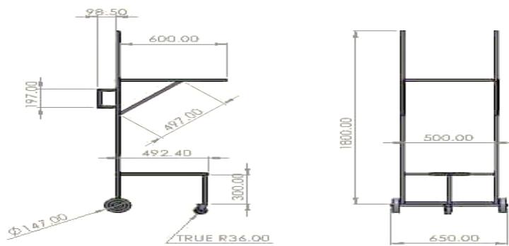
ภาพที่ 5 การออกแบบรถเข็นขนย้ายเก้าอี้
