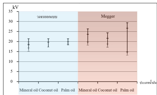
รูปที่ 4 กราฟแสดงผลการเปรียบเทียบค่าแรงดันเบรคดาวน์ของน้ำมัน 3 ประเภทด้วยวงจรออกแบบและเครื่องมือมาตรฐาน
