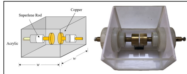
รูปที่ 2 อิเล็กโทรดที่ได้ออกแบบไว้
