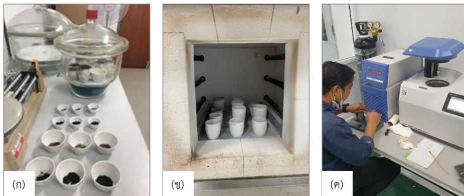
ภาพที่ 3 การเตรียมตัวอย่างวัตถุดิบเพื่อทดสอบสมบัติทางเคมี โดยการทดสอบหาปริมาณความชื้น (ก) นำตัวอย่างเข้าเตาเผาอุณหภูมิสูงเพื่อหาปริมาณเถ้า ปริมาณสารระเหย และปริมาณคาร์บอนคงตัว (ข) และหาค่าพลังงานความร้อนจากเครื่อง bomb calorimeter (ค)
